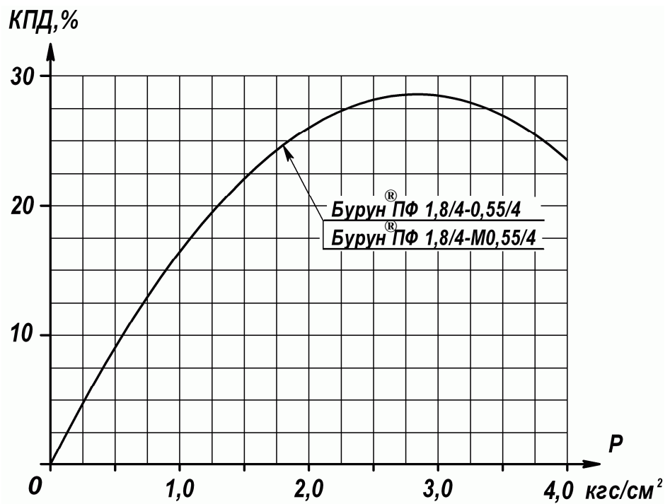
Рисунок 2- Характеристика электронасосов
